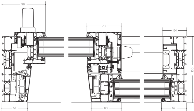
Horisontellt tvärsnitt 1 skjutbar del + fast del
