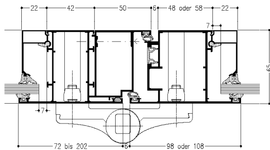
Anschlagtür nach außen öffnend
