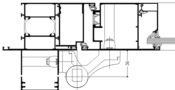
Aluminium Aufsraubband Dr. Hahn
