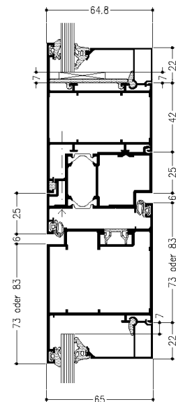
Anschlagtür nach innen öffnend mit Oberlicht
