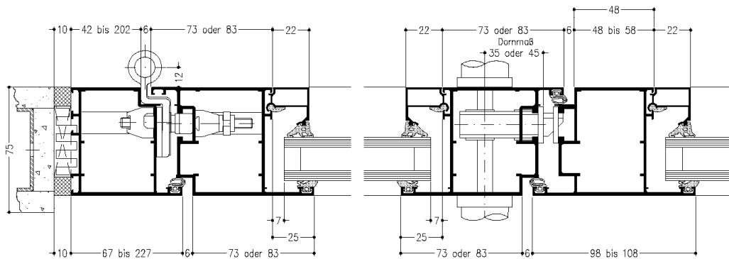
Anschlagtür nach innen öffnend mit Alu-Rollenband Typ WICONA
