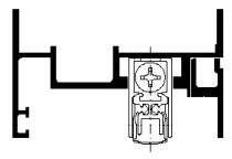
Tür auswärts Umlaufender Flügel
