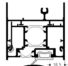
Tür auswärts Sockellösung
