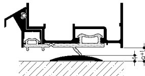
Tür einwärts Umlaufender Flügel
