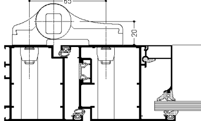
Aluminium Aufschraubband Dr. Hahn
