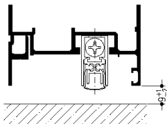
Tür einwärts Umlaufender Flügel
