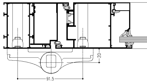
Aluminium Aufsraubband Dr. Hahn
