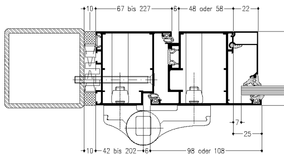
Anschlagtür nach außen öffnend mit Alu-Aufschraubband Typ Dr. Hahn
