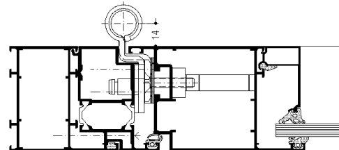
Edelstahl-Rollenband WICONA
