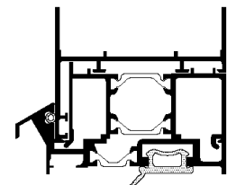
Tür auswärts Sockellösung
