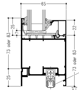
Anschlagtür nach innen öffnend mit umlaufendem Flügel und Absenkdichtung
