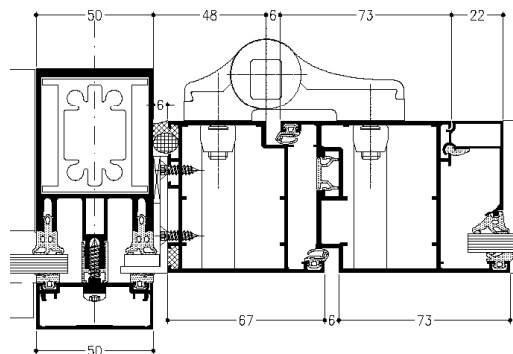
Anschlagtür nach innen öffnend Einbau in Fassade
