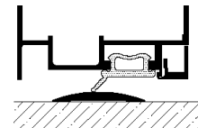
Tür auswärts Umlaufender Flügel
