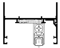
Tür einwärts oder auswärts Kämpfer als Sockel
