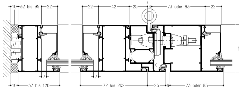
Anschlagtür nach innen öffnend mit Seitenteil
