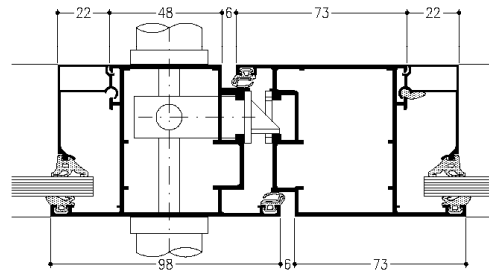
Anschlagtür nach außen öffnend Mittelstoß
