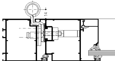
Edelstahl-Rollenband WICONA
