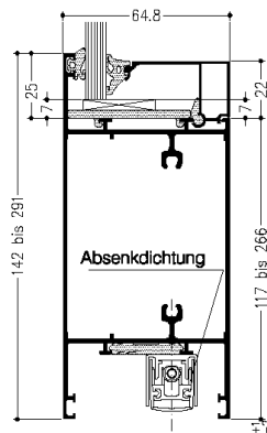
Anschlagtür nach außen öffnend mit Sockel und Absenkdichtung
