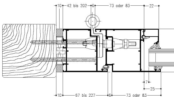
Anschlagtür nach innen öffnend mit Alu-Rollenband Typ WICONA
