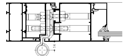
Edelstahl-Rollenbandband WICONA
