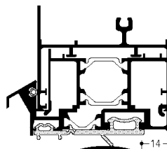
Tür einwärts Sockellösung
