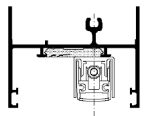
Tür einwärts oder auswärts Sockellösung
