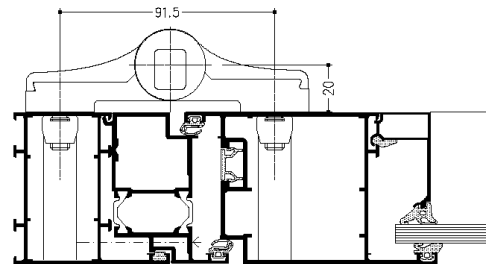
Aluminium Aufschraubband Dr. Hahn
