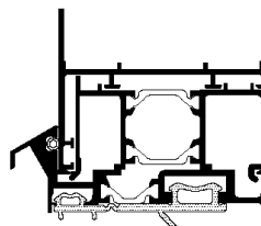
Tür einwärts Sockellösung
