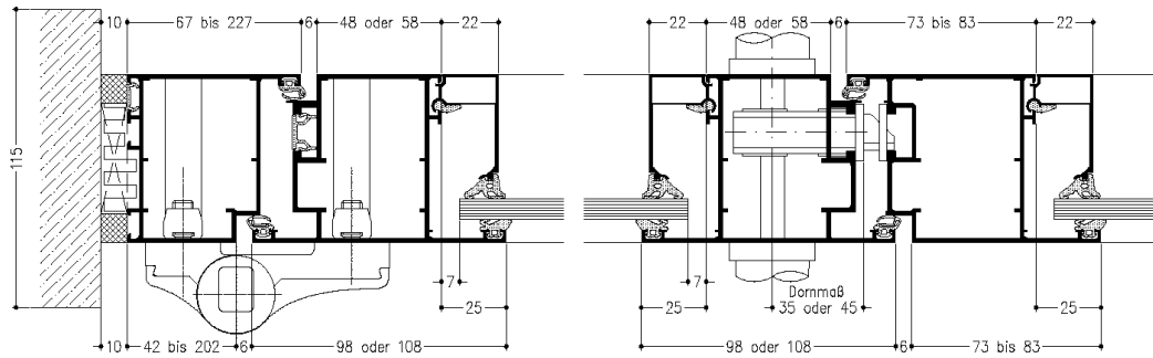
Anschlagtür nach außen öffnend mit Alu-Aufschraubband Typ Dr. Hahn
