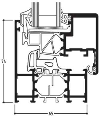
Coupe verticale (échelle 1/2)
