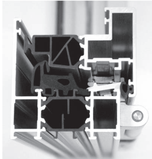
Ouvrant caché Wicline 65 HI
