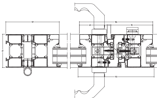
Sección horizontal
